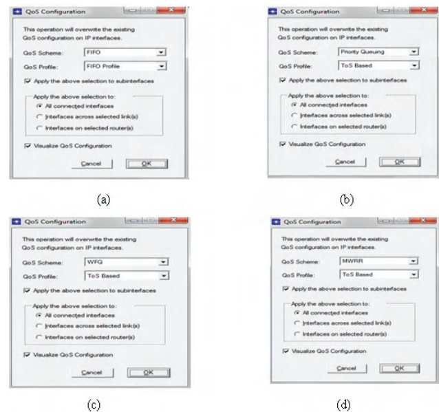
Fig. 2. Router configuration for (a) FIFO (b) PQ (c) WFQ (d) MWRR
