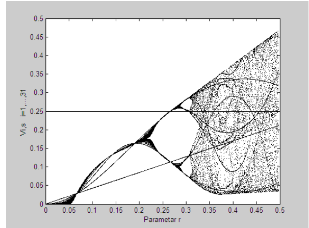
Fig. 9a. Bifurcation diagram
