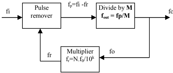
Fig.3. Basic Fractional-N.
