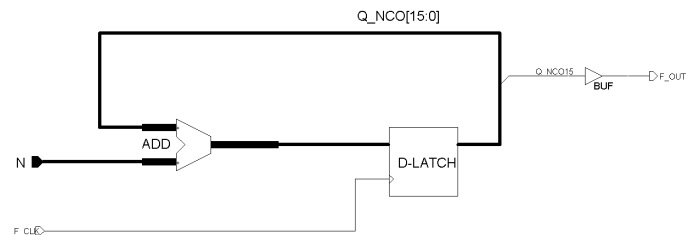
Fig. 4. DCO.
