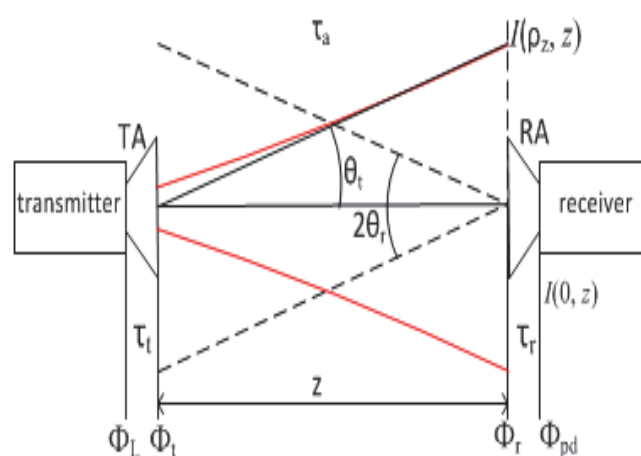
Fig. 1. FSO link and system parameters
